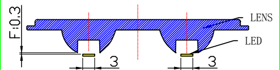
光学装配示意图
