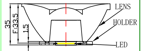
光学装配视图
