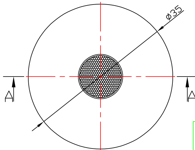
光学装配视图
