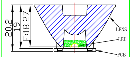
光学装配视图
