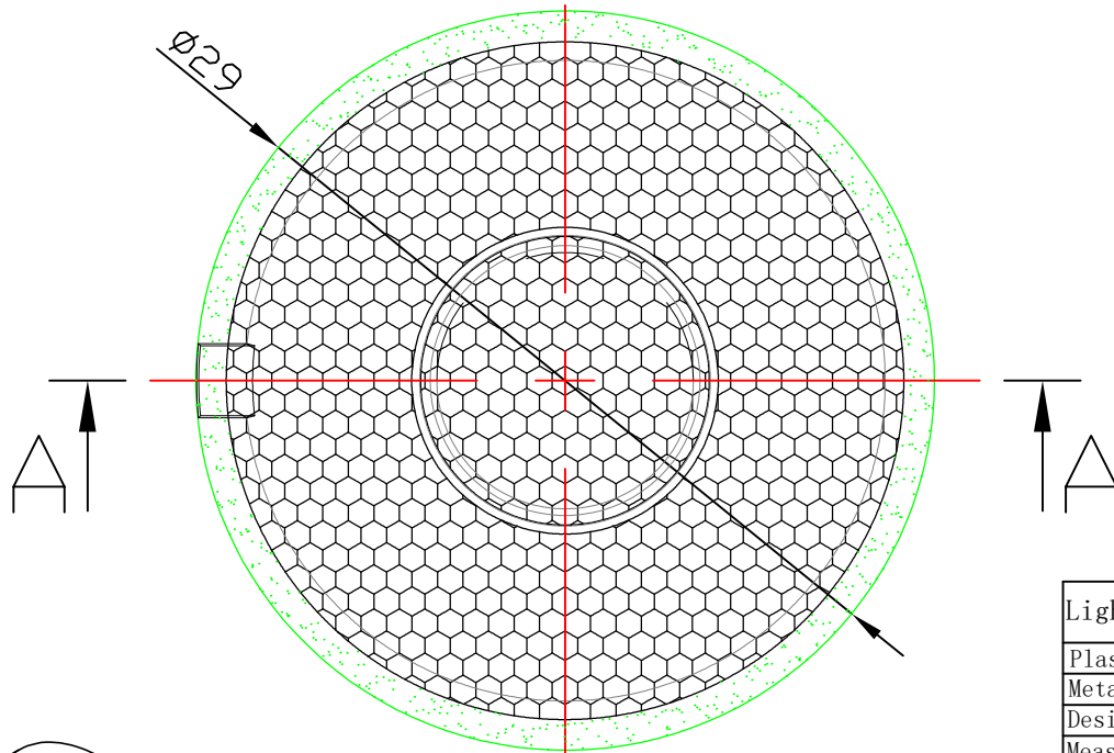
光学装配示意图
