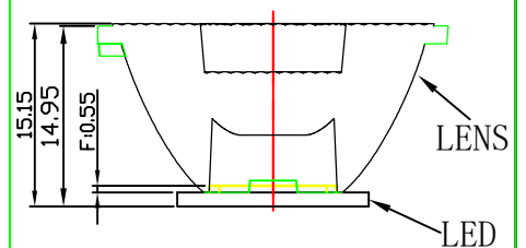
光学装配示意图
