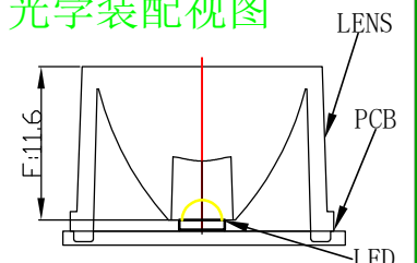
光学装配视图
