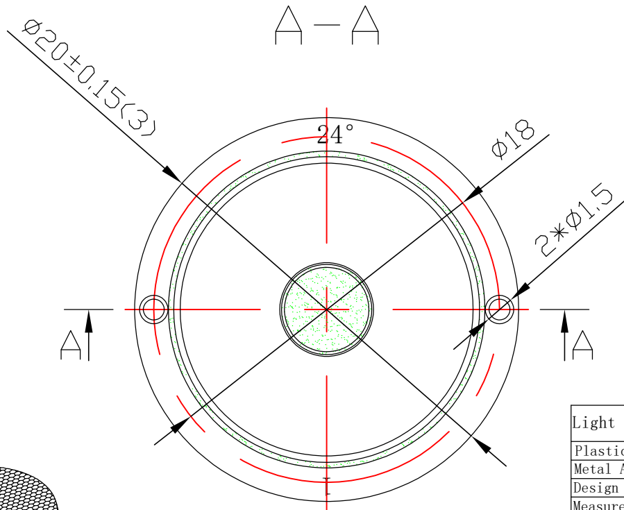
光学装配视图
