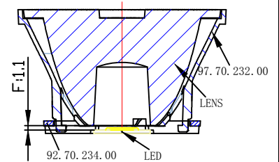
光学装配示意图
