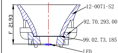
光学装配示意图
