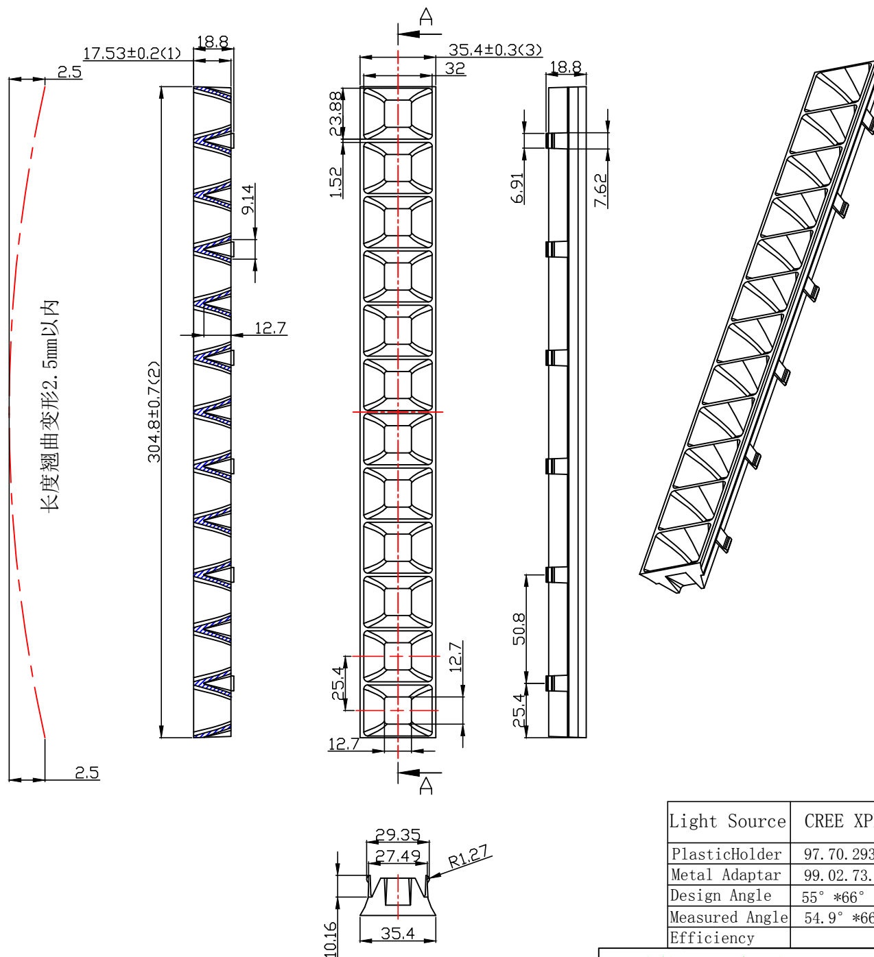
光学装配示意图
