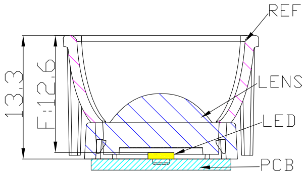
光学装配示意图
