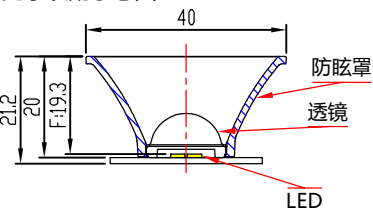
光学装配示意图
