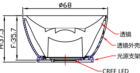
光学装配示意图
