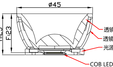
光学装配示意图
