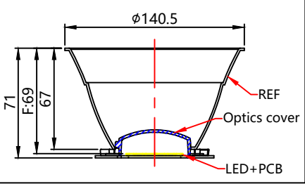
光学装配示意图
