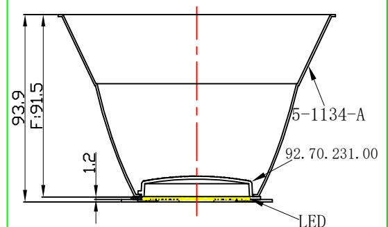
光学装配示意图
