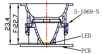
光学装配示意图
