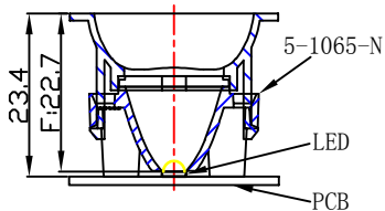
光学装配示意图
