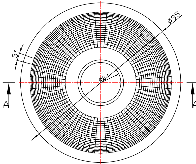
光学装配示意图
