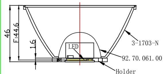
光学装配示意图
