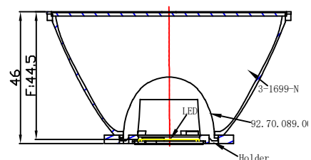
光学装配示意图
