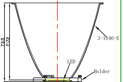
光学装配示意图
