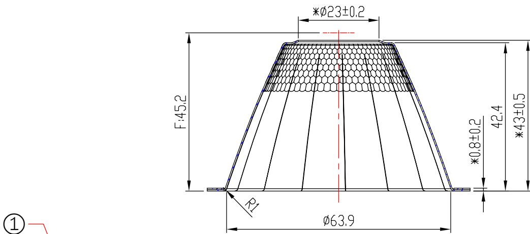
A-A
