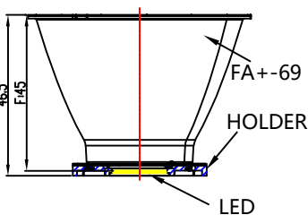
光学装配示意图
