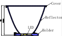
光学装配示意图
