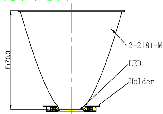
光学示意图
