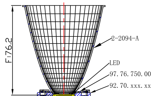
光学示意图
