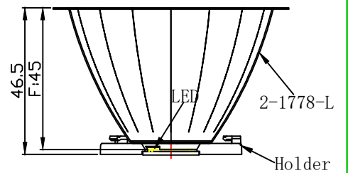
光学装配示意图
