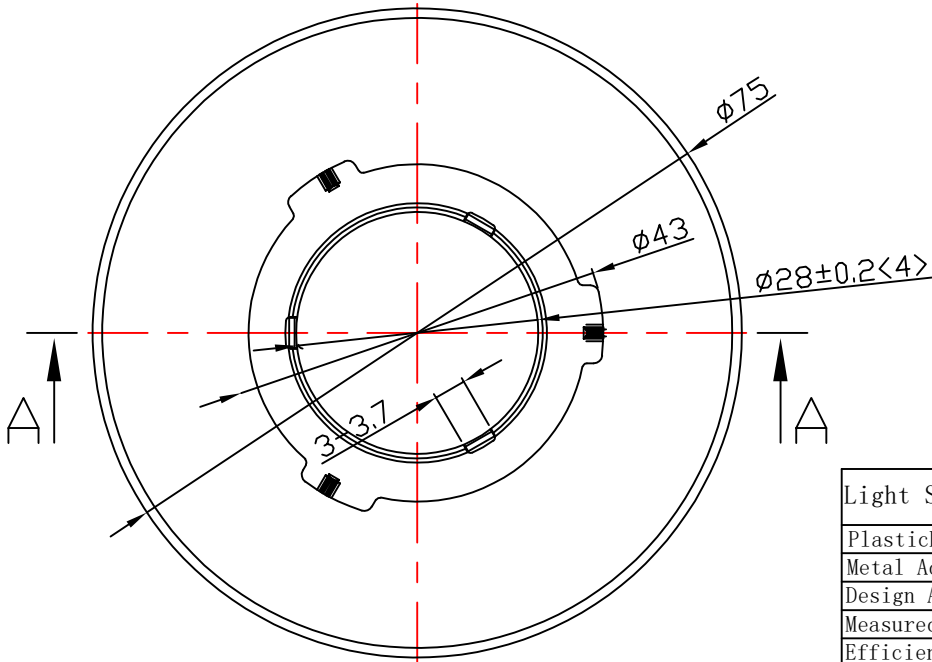
光学装配示意图
