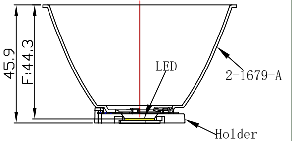
光学装配示意图
