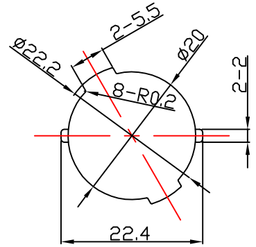
底孔视图 1:1
