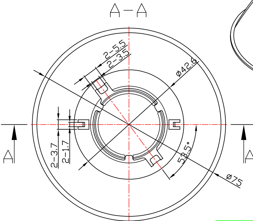
光学装配示意图
