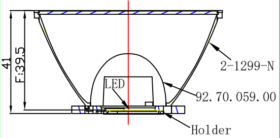
光学装配示意图
