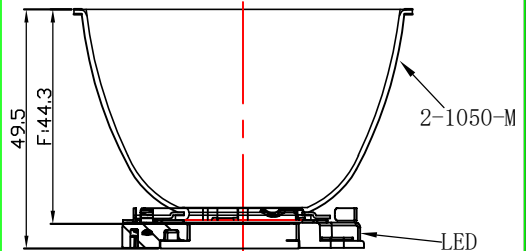
光学装配示意图
