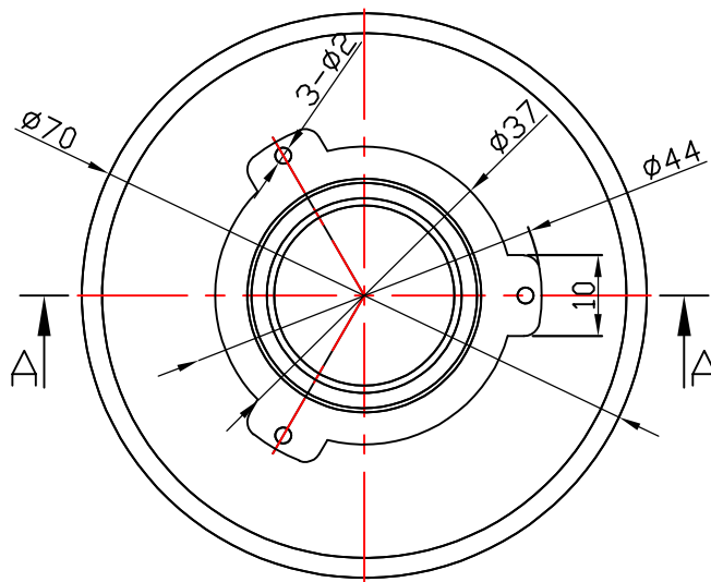
光学装配示意图
