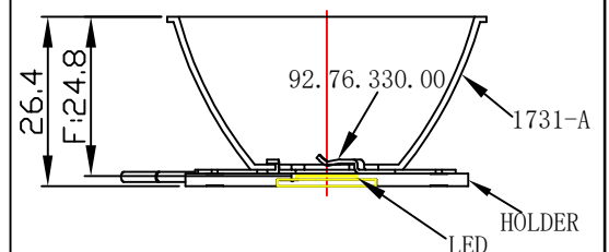
光学装配示意图
