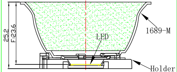
光学装配示意图
