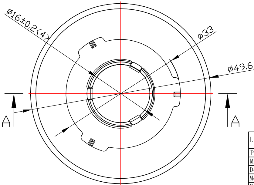
光学装配示意图
