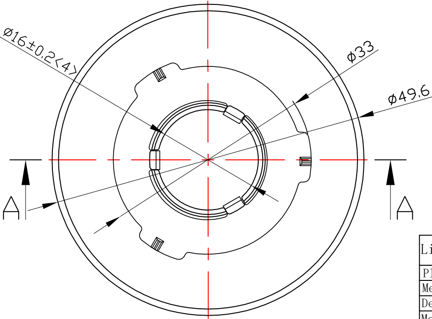
光学装配示意图
