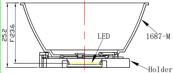
光学装配示意图
