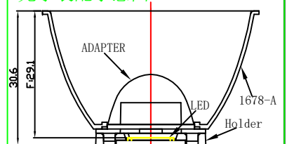
光学装配示意图
