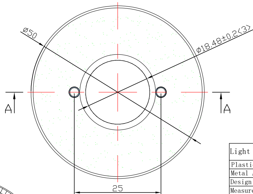
光学装配示意图
