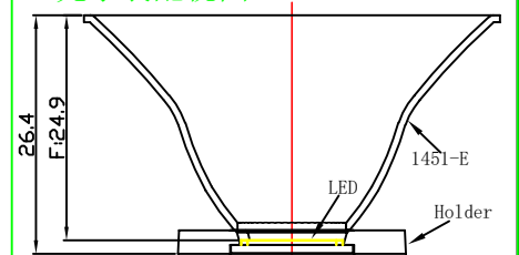
光学装配视图
