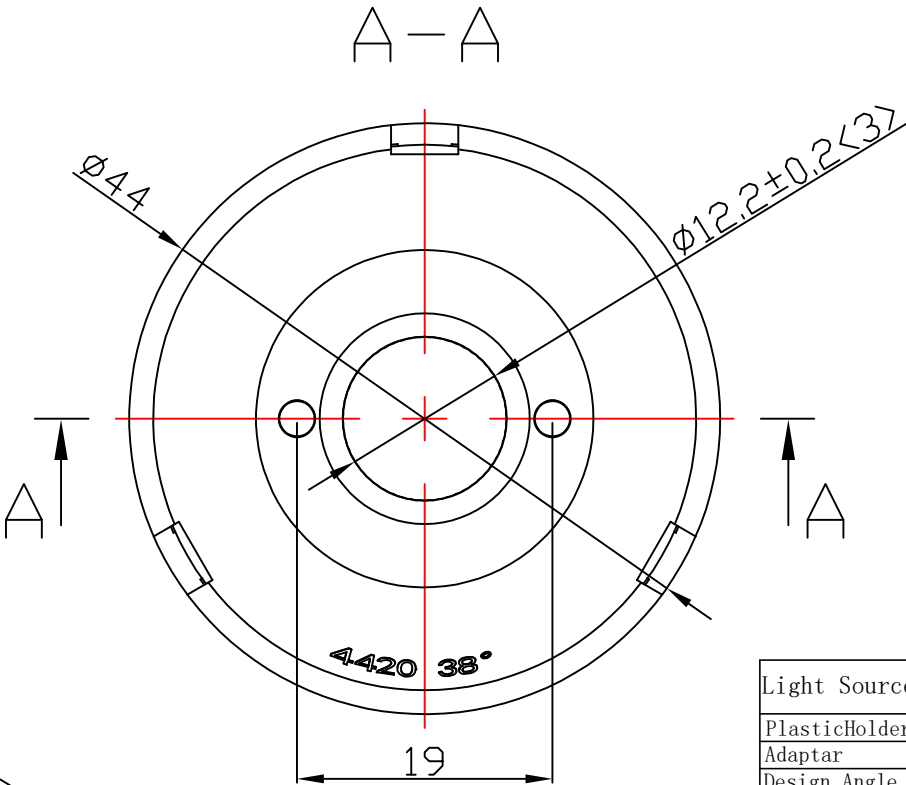
光学装配示意图
