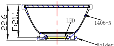
光学装配示意图
