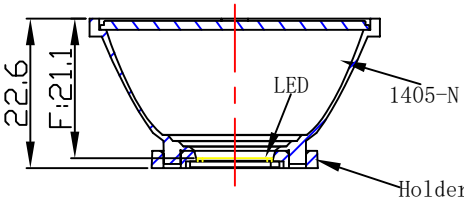
光学装配示意图
