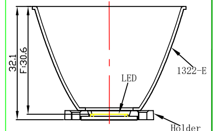
光学装配示意图
