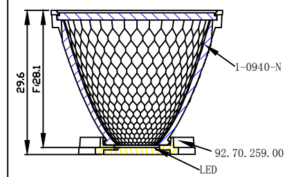
光学装配示意图
