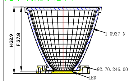
光学装配示意图
