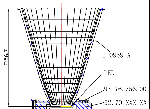
光学示意图
