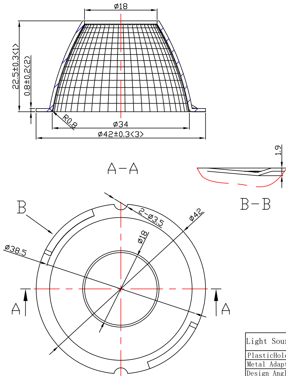
光学装配示意图
