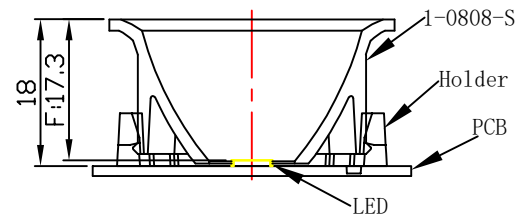
光学装配示意图
