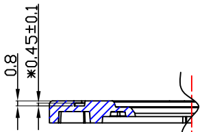
C-C 1:1
