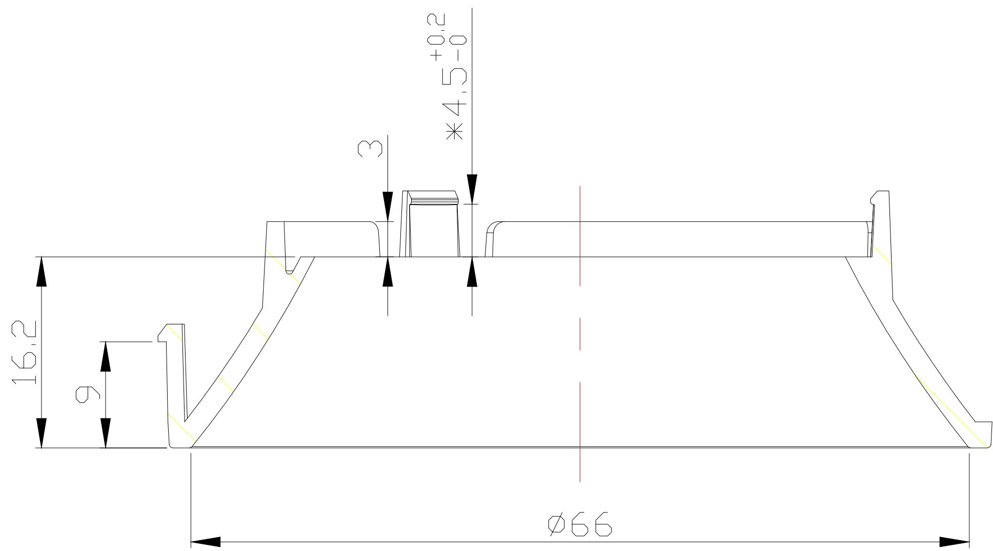
A-A
